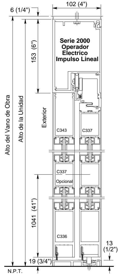
Escala : 1:4 (3" = 1'-0") Puerta mostrada en posición abierta.
