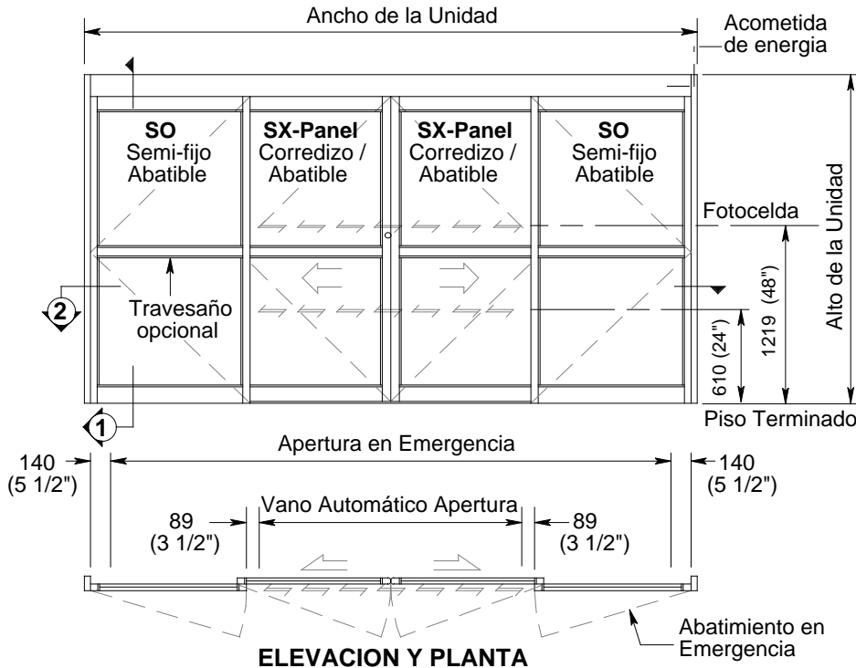
Escala: 1:50 (1/4" = 1'-0") 4267 (14'-0") ancho unidad mostrada
