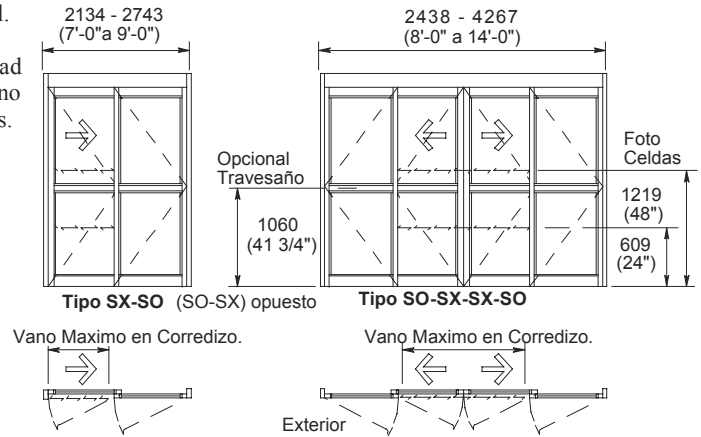
Elevaciones y Plantas Arquitectonicas
