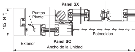
Seccion Horizontal
